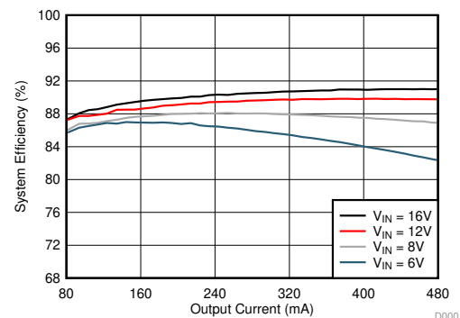
系统效率
