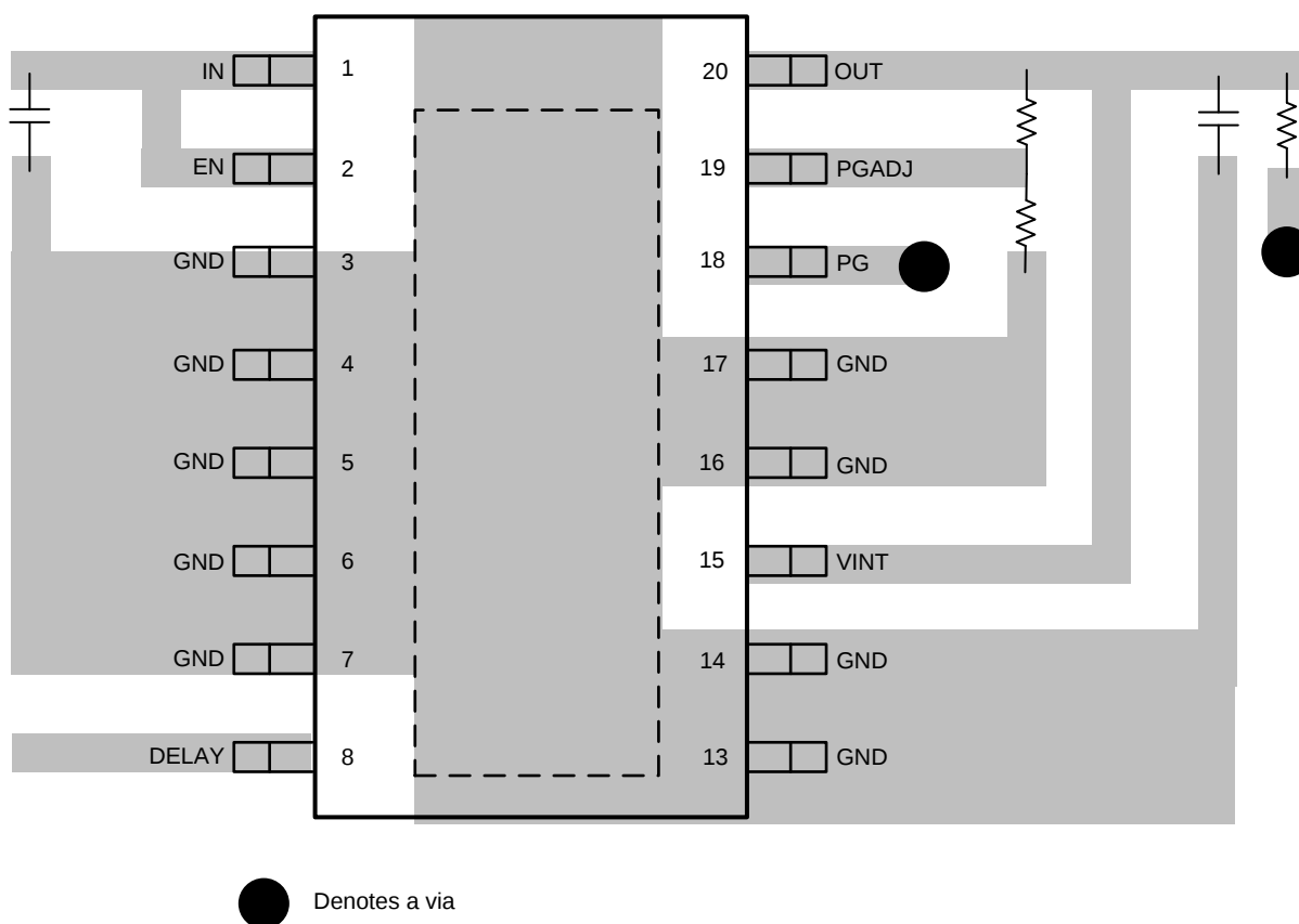
图 25. Layout Example
