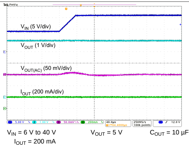
图 17. Line Transient
