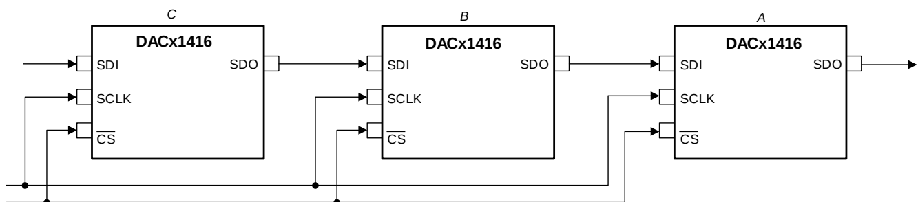
图 51. Daisy-Chain Layout
