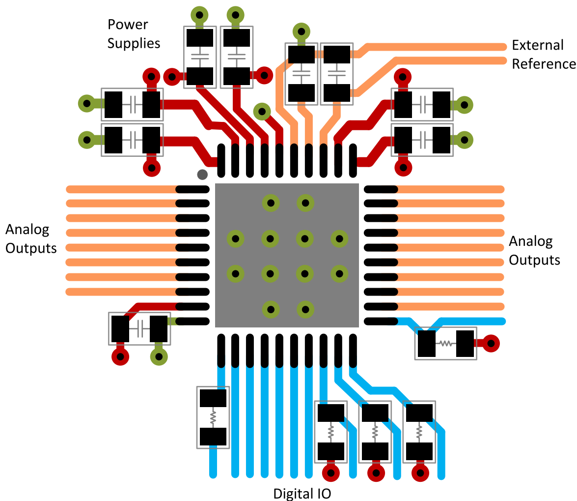
图 70. Example Layout
