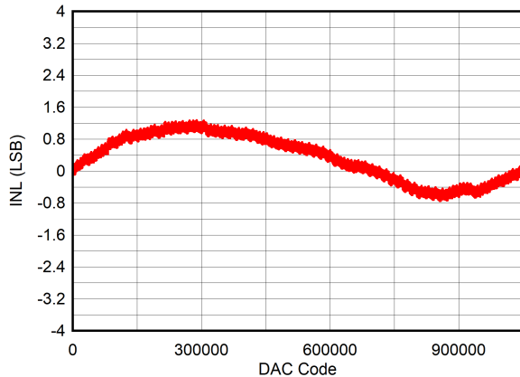
图 57. INL at \pm 10 -V Output
