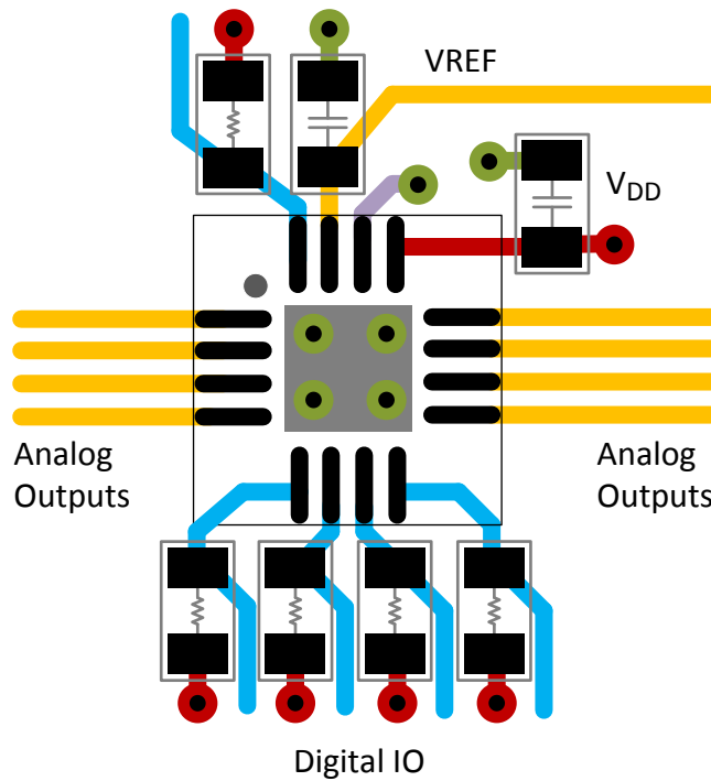
图 68. 布局示例
