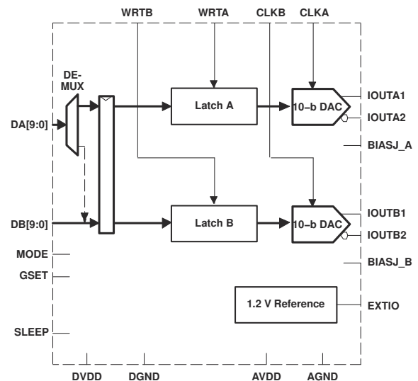
功能方框图
