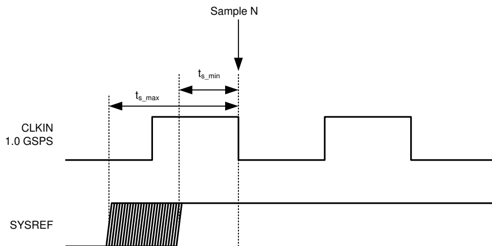
图 7-1. SYSREF Timing
