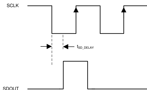
图 8-18. SDOUT Timing Diagram
