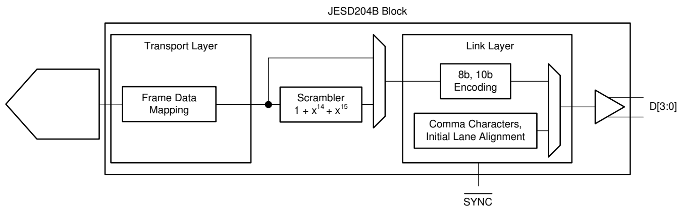
图 8-20. JESD204B Transmitter Block
