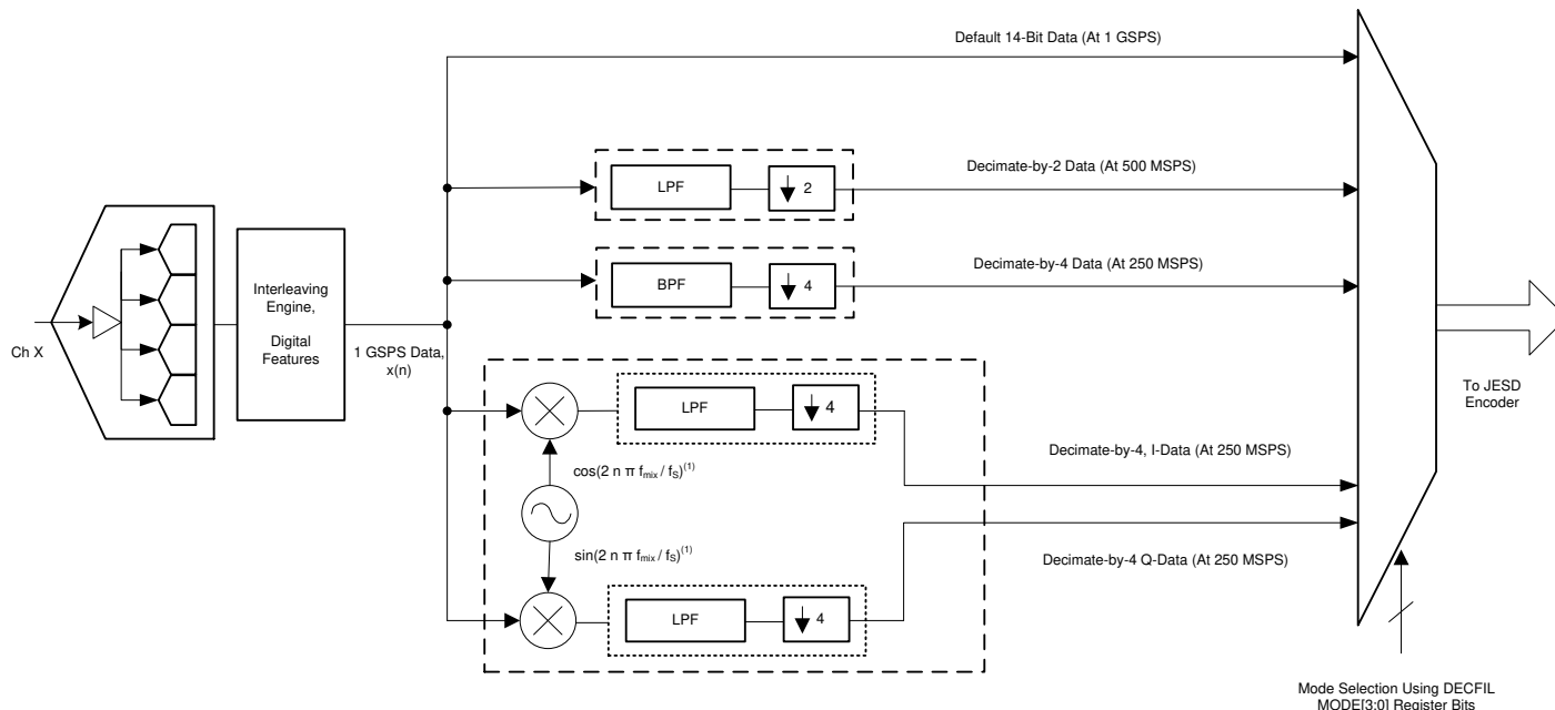
图 8-3. DDC Block
