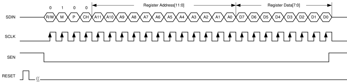
图 8-15. SPI Page Selection
