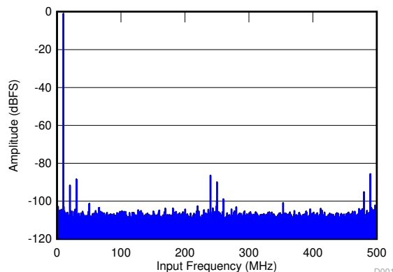
图 7-3. FFT for 10-MHz Input Signal
