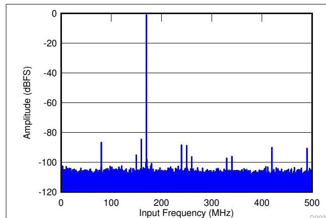
图 9-18. FFT for 170-MHz Input Signal
