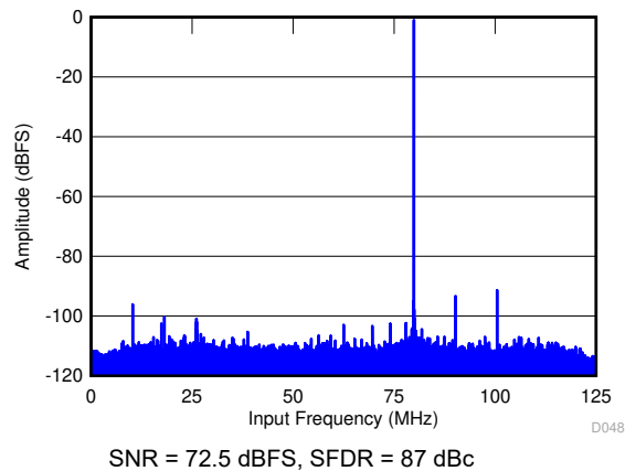
图 7-51. FFT for 170-MHz Input Signal in Decimate-by-4 Mode
