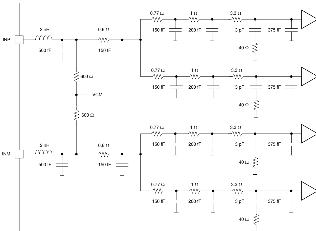
图 8-1. Analog Input Network
