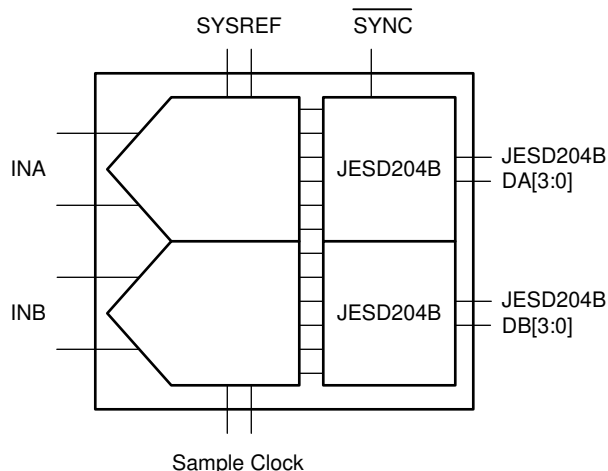
图 8-19. ADS54J40 Block Diagram
