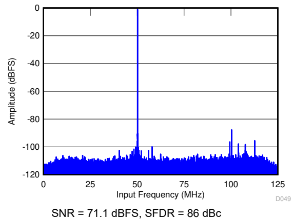
图 7-52. FFT for 300-MHz Input Signal in Decimate-by-4 Mode
