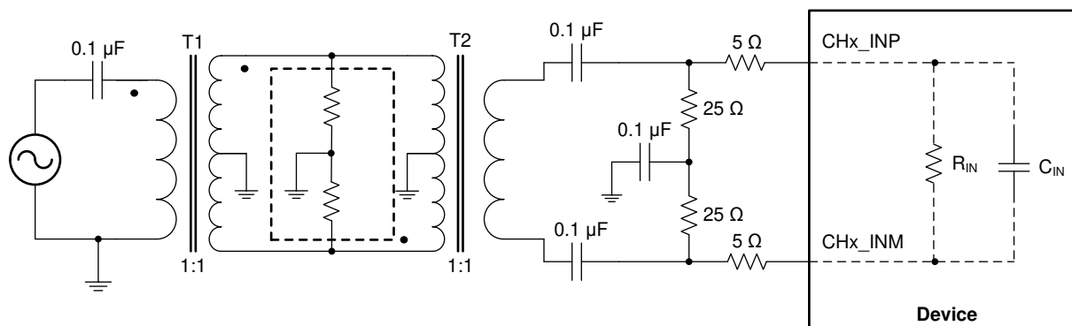
图 9-17. Input Drive Circuit
