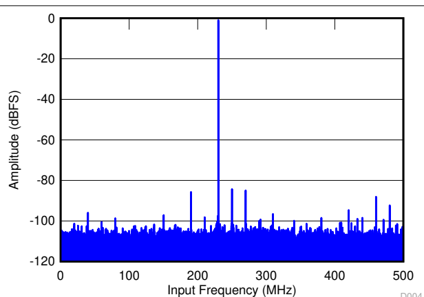
图 9-19. FFT for 230-MHz Input Signal
