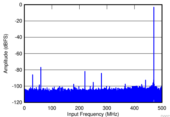
图 7-9. FFT for 470-MHz Input Signal at - 3 dBFS
