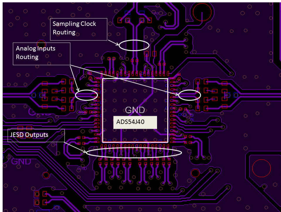
图 11-1. ADS54J40 EVM Layout
