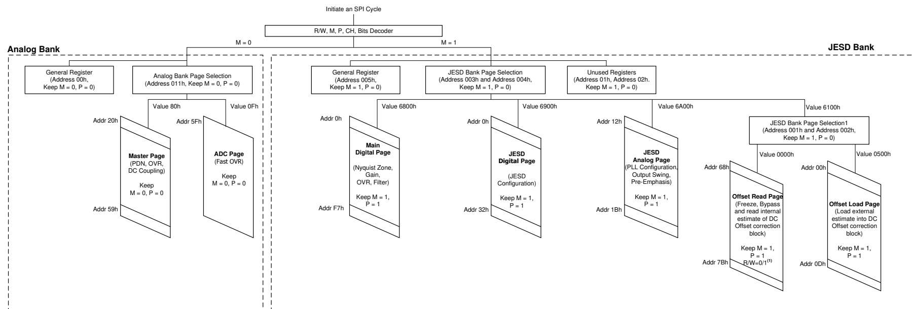
图 8-27. Serial Interface Registers
