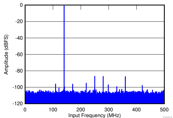
图 7-4. FFT for 140-MHz Input Signal
