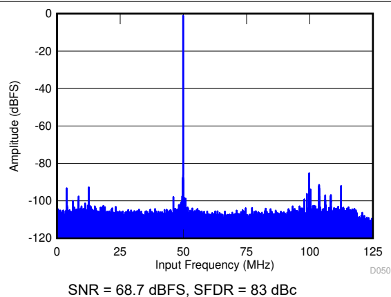
图 7-53. FFT for 450-MHz Input Signal in Decimate-by-4 Mode
