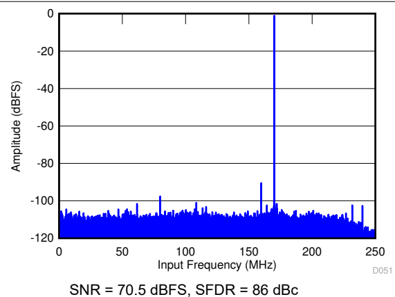
图 7-54. FFT for 170-MHz Input Signal in Decimate-by-2 Mode
