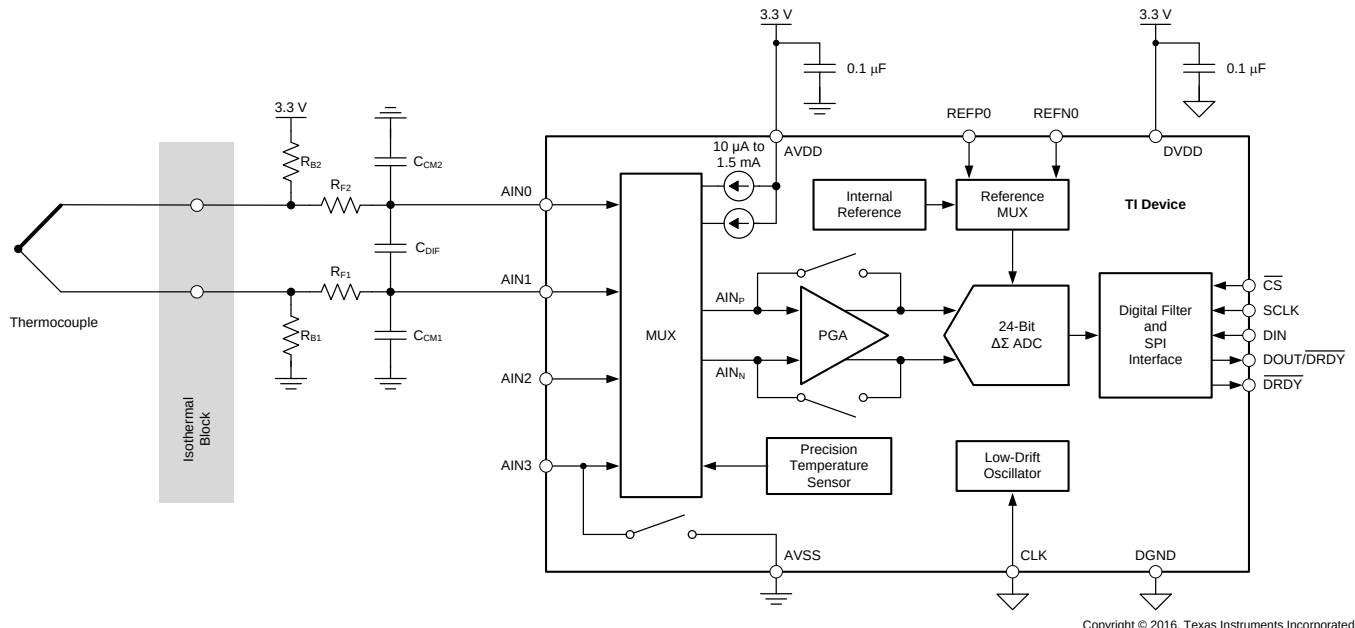
图 74. 热电偶测量
