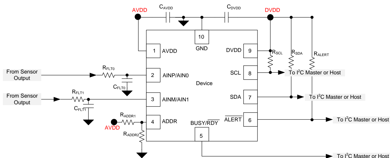
图 123. Example Circuit
