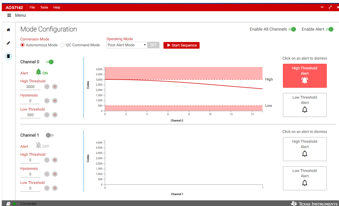
图 118. Post Alert Data Capture
