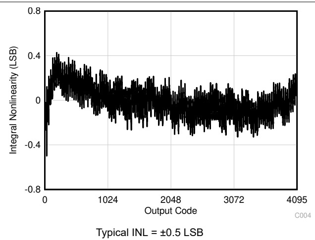
图 7-6. Typical INL
