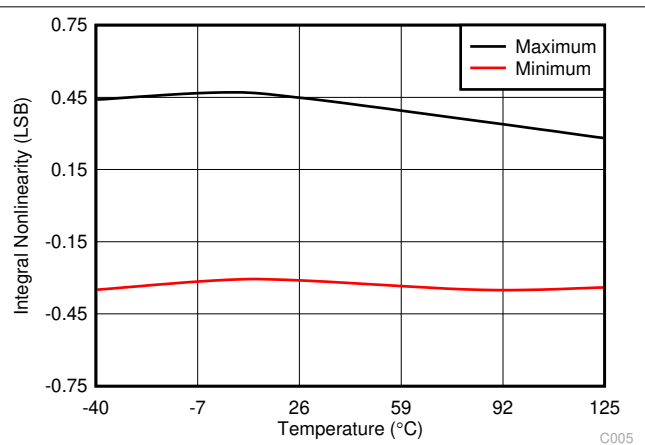
图 7-6. Typical INL
