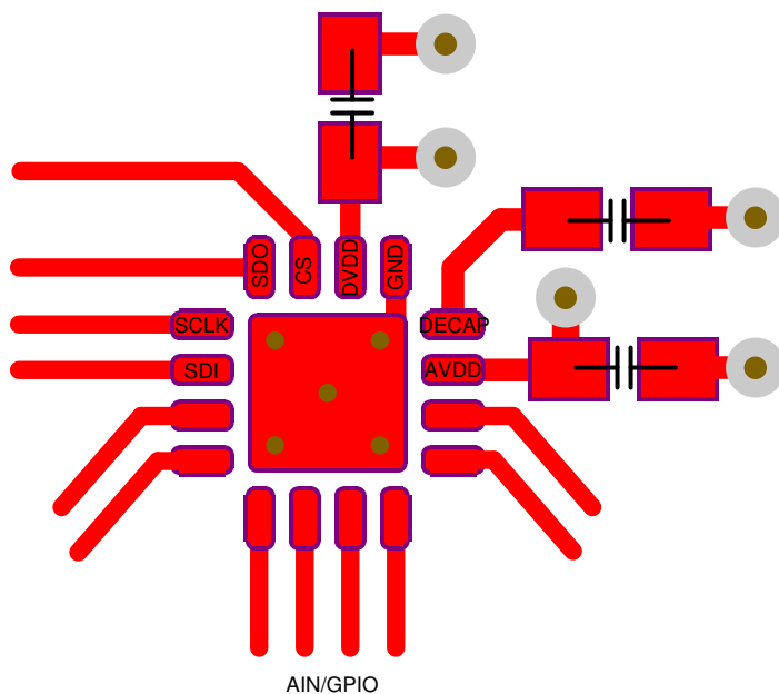
图 11-1. Example Layout
