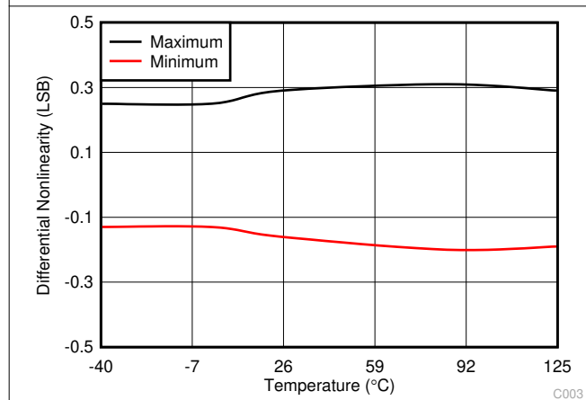
图 7-5. Typical DNL
