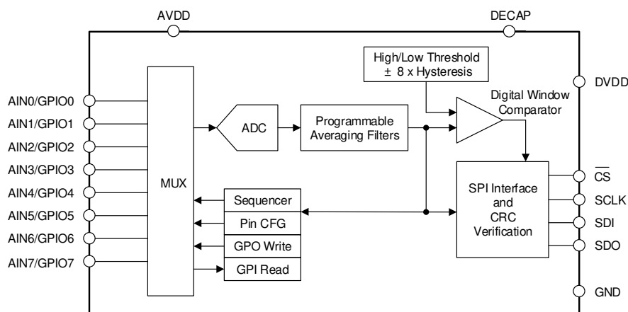
ADS7038-Q1 方框图和应用
