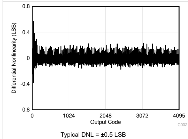
图 7-5. Typical DNL
