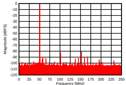
–1dBFS、450MHz 输入时的频谱
