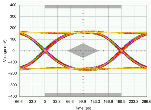
18 英寸、5 密耳输出端的传输眼图。 5Gb/s、 带优化型去加重功能的 FR4 微带迹线
