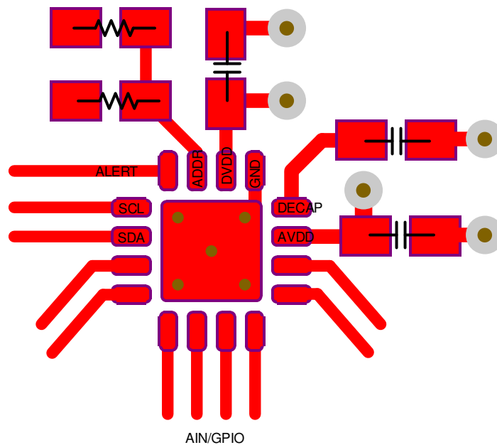
图 11-1. Example Layout
