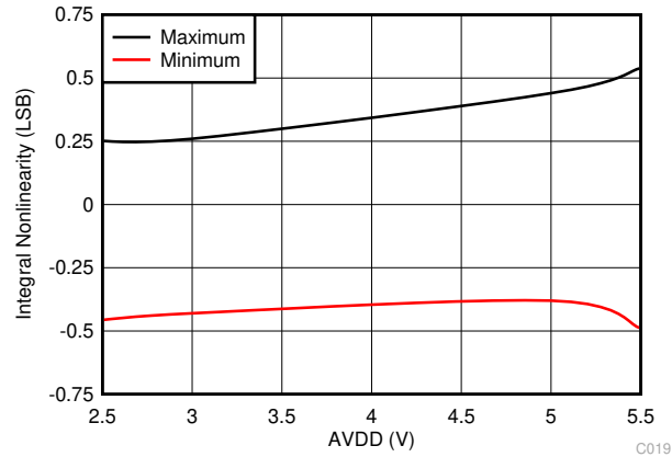
图 7-8. INL vs AVDD
