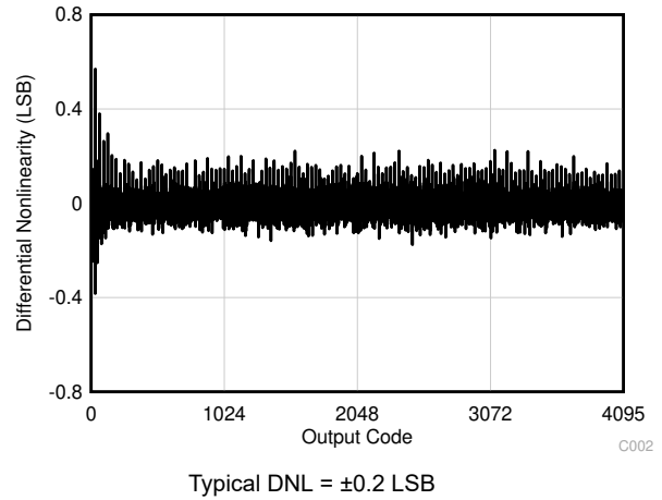
图 7-3. Typical DNL
