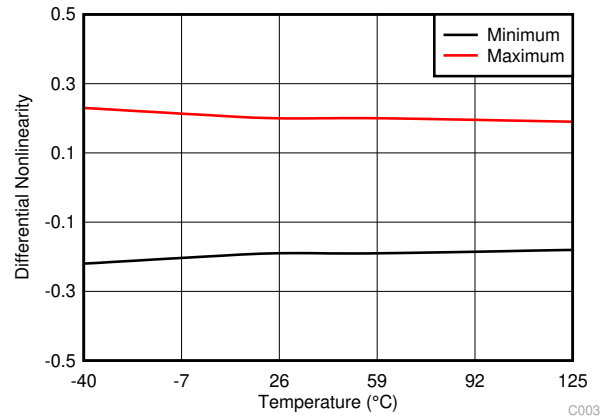
图 7-3. Typical DNL
