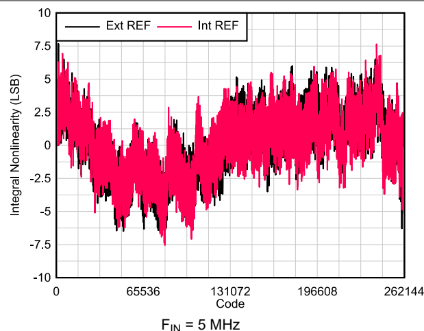
图 6-21. INL vs Code
