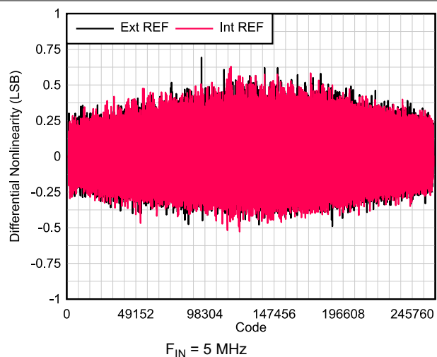
图 6-22. DNL vs Code
