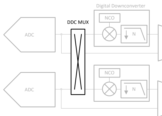
图 8-20. DDC MUX
