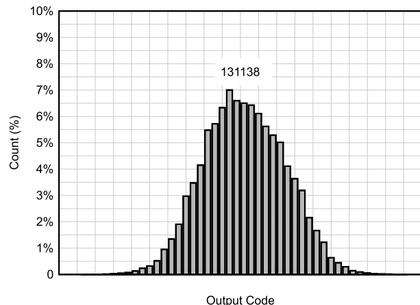
图 6-23. DC Offset Histogram
