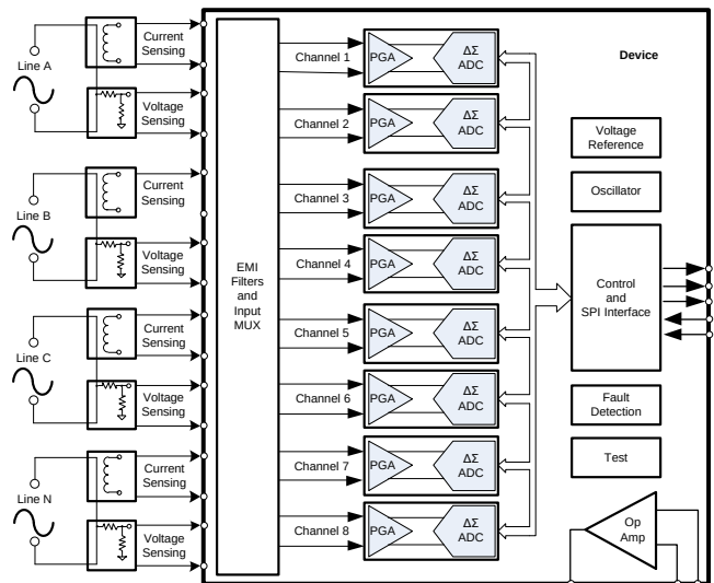
ADS131E08 简化电路原理图
