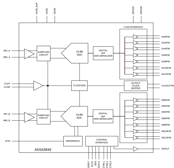
框图
