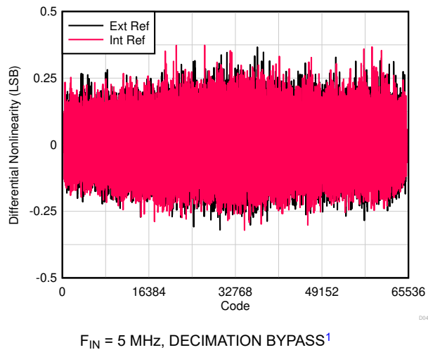
图 6-21. DNL vs Code
