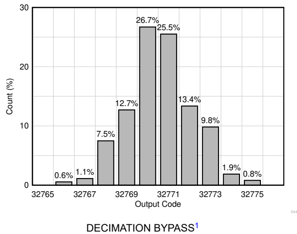
图 6-19. DC Offset Histogramm
