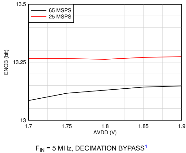
图 6-17. ENOB vs AVDD
