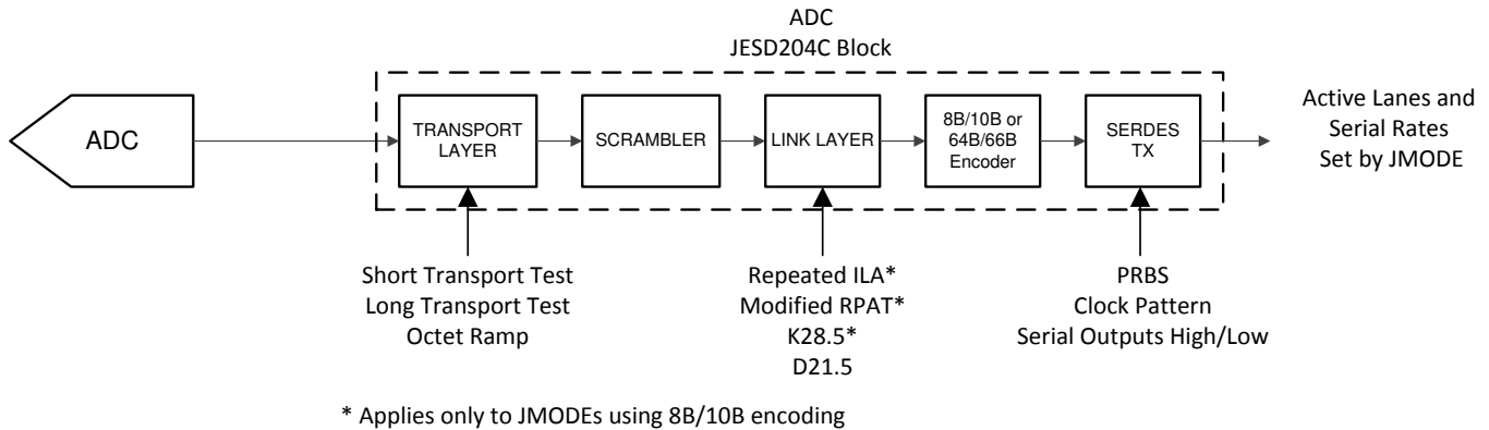
图 12. Test Mode Insertion Points
