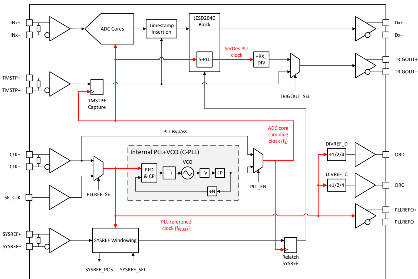
图 5. ADC12QJ1600-Q1 Clocking Subsystem
