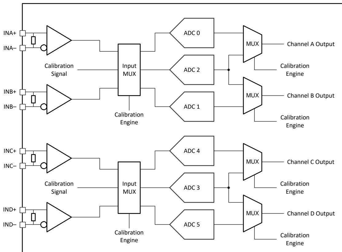
图 13. ADC12QJ1600-Q1 Calibration System Block Diagram
