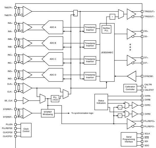
ADC12QJ1600-Q1 方框图
