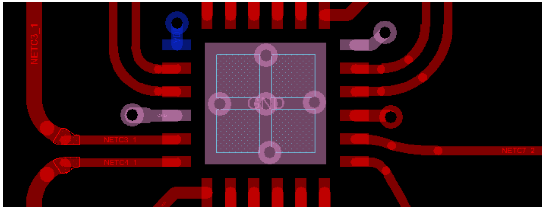
图 30. Example Layout
