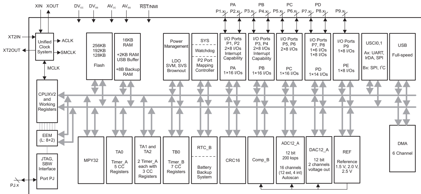
图 1-1. 功能框图 – MSP430F5638、MSP430F5637 和 MSP430F5636
