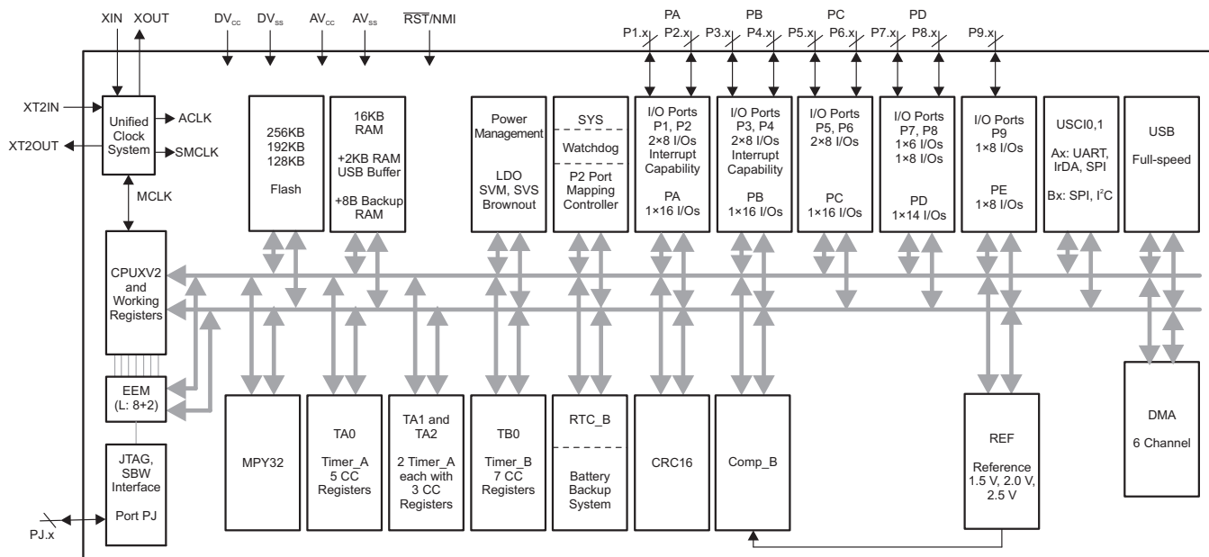
图 1-3. 功能框图 – MSP430F5632、MSP430F5631 和 MSP430F5630
