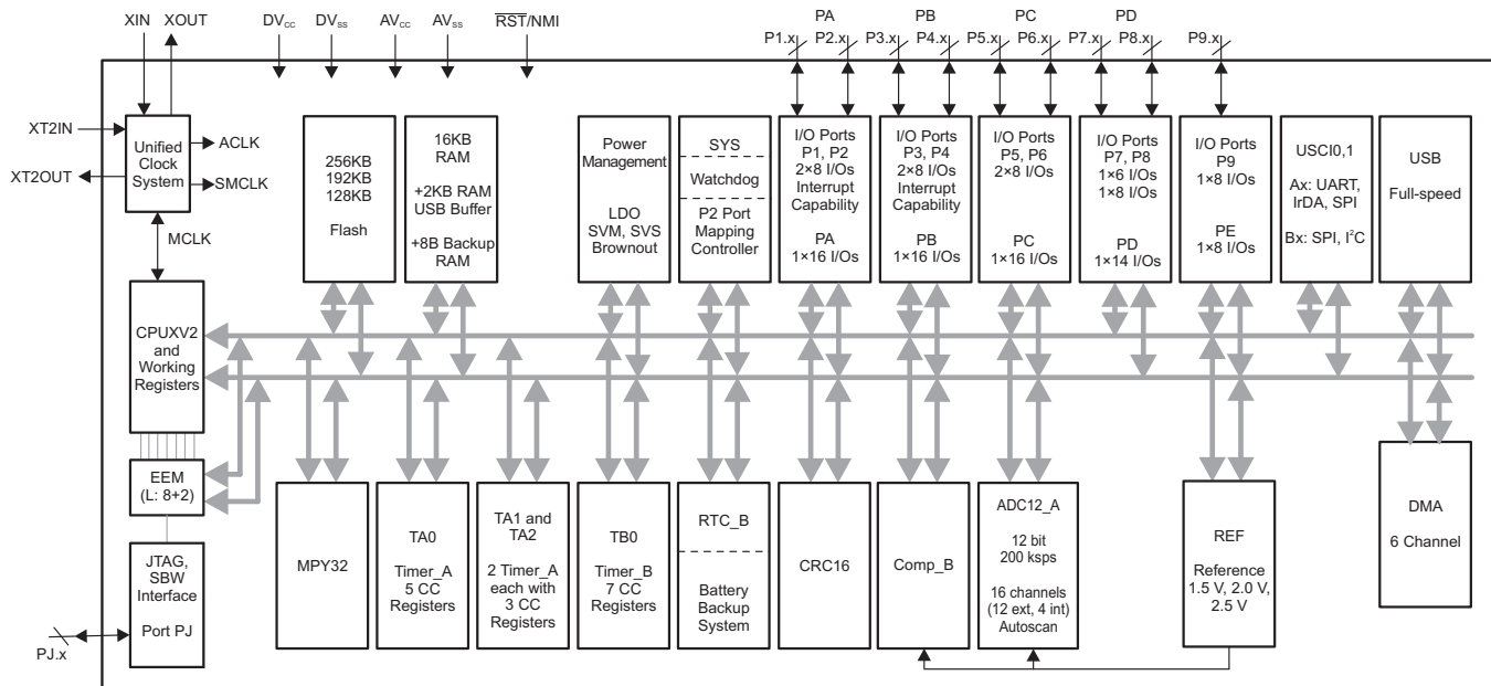
图 1-2. 功能框图 – MSP430F5635、MSP430F5634 和 MSP430F5633
