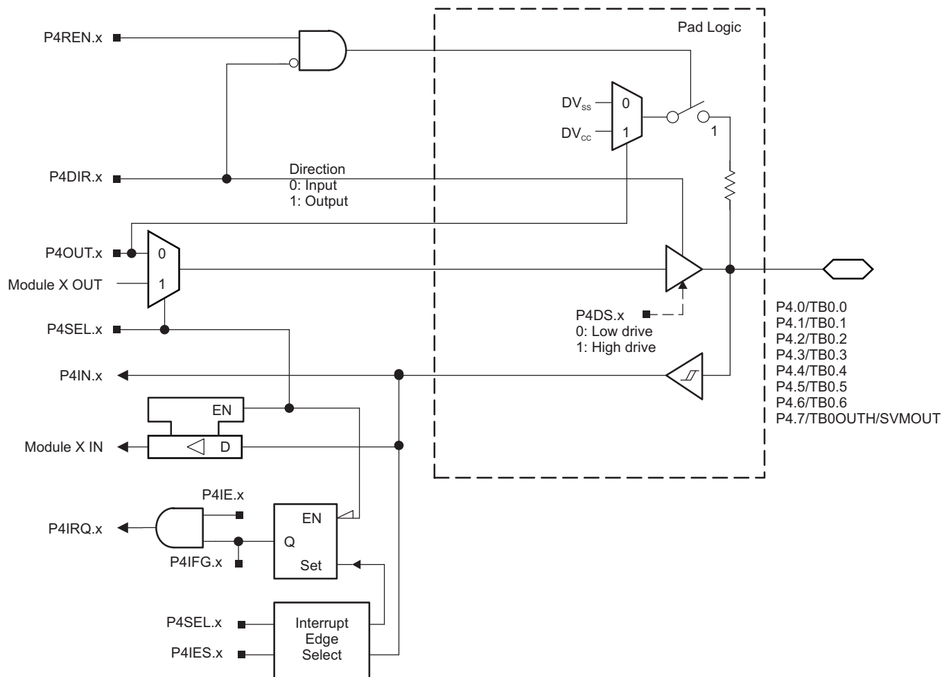
图 6-5. Port P4 (P4.0 to P4.7) Diagram
