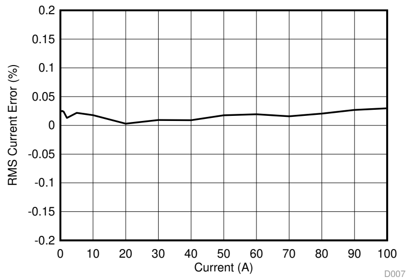
图 94. Phase B RMS Current % Error
