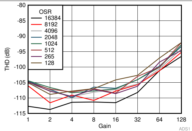
图 17. THD vs Gain
