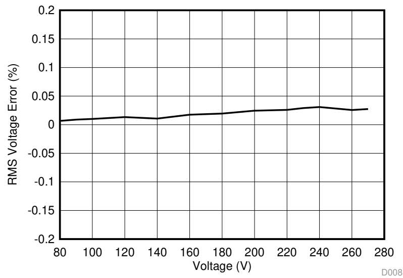
图 95. Phase A RMS Voltage % Error
