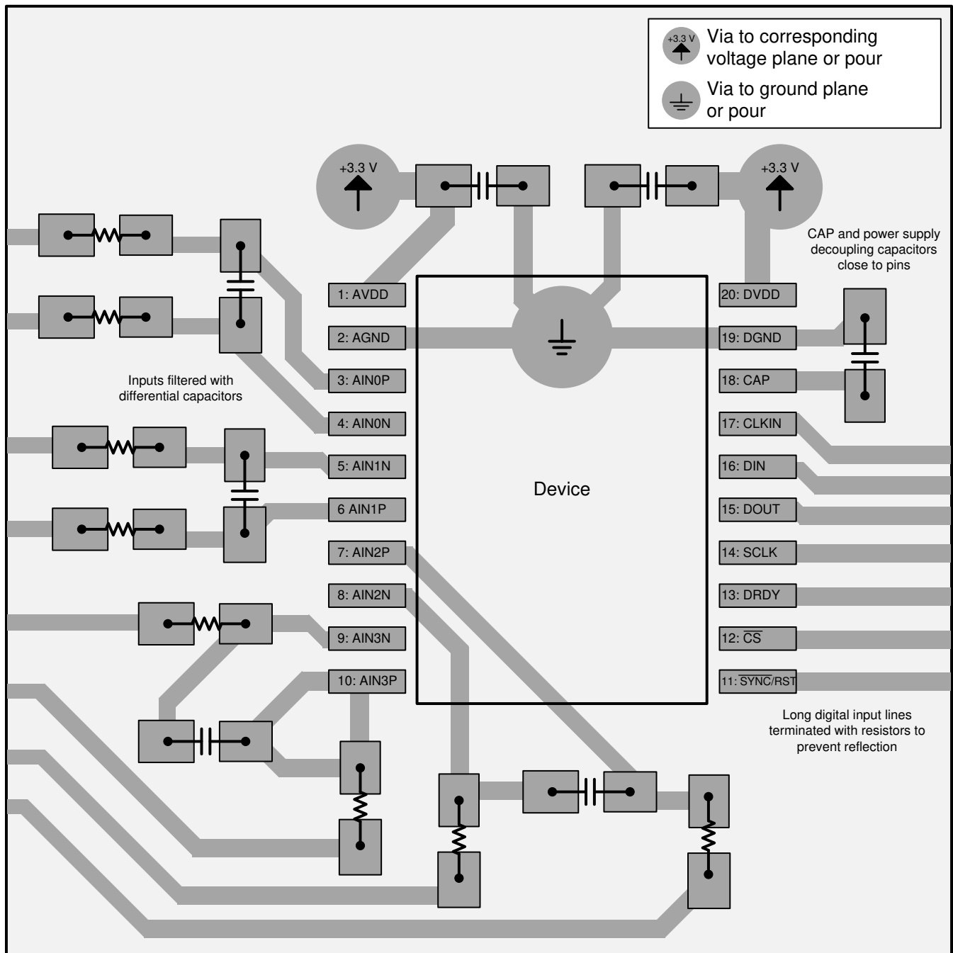
图 97. Layout Example
