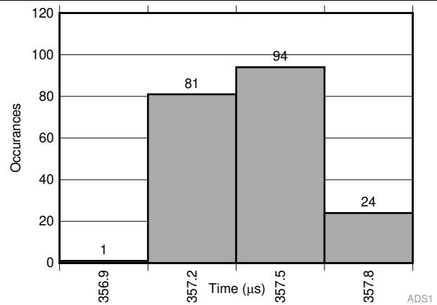
图 5. Startup Time Histogram
