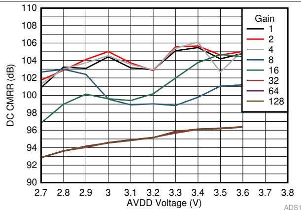
图 10. DC CMRR vs AVDD
