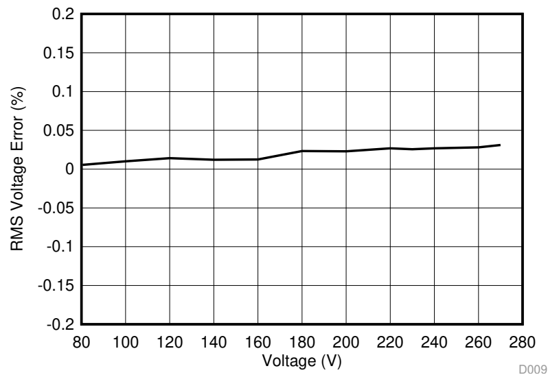
图 96. Phase B RMS Voltage % Error
