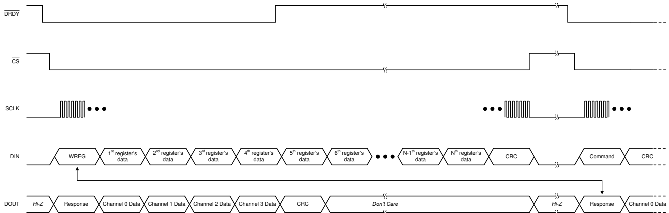
图 47. Writing Registers
