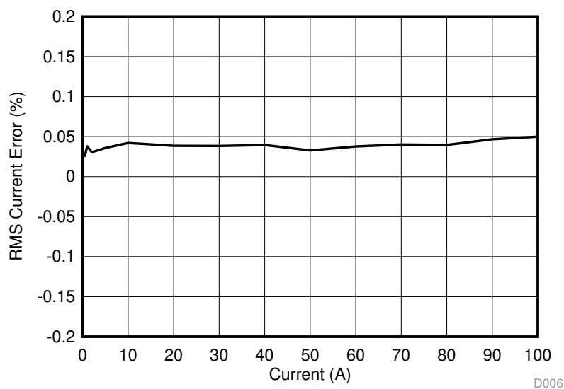
图 93. Phase A RMS Current % Error
