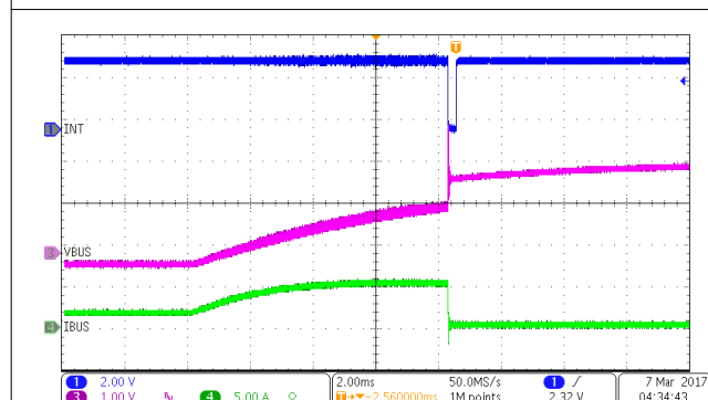
Figure 10-4. VBUS_OVP
