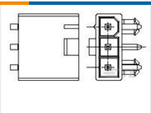
TE 产品编号2029150-5 5P R/A HDR VAL-U-LOK V2 W/P
