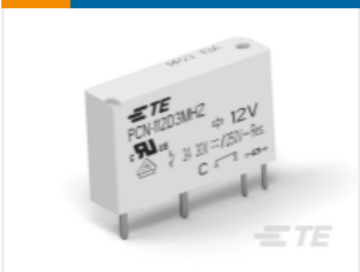
TE 产品编号1721547-7 PCN 3A/5A 纤薄 PCB 继电器 3VDC
