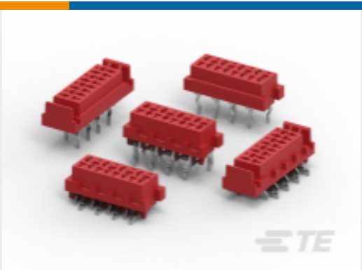
TE 产品编号1-338069-8 板母端连接器顶端插入
