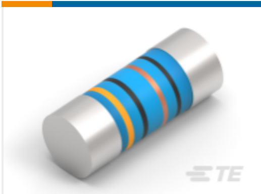
TE 产品编号1-2176316-4 MELF SMA_A 1K2 0.1% 15PPM 0207 1W
