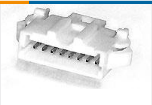
TE 产品编号1-292215-8 MINI CT SGL RELAY 18P NAT
