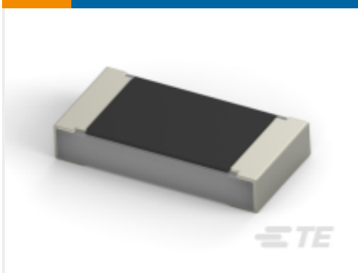
TE 产品编号2-2176230-8 SMD 功率电阻器：3 瓦特，5% Tol
