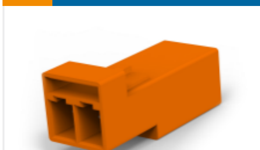
TE 产品编号1-2834049-4 LIGHT-N-LOK 模块化锁闭母端
