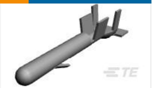
TE 产品编号61118-7 CMNL PIN 20-14 AUNIBR
