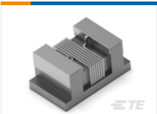
TE 产品编号1879591-9 3650 0402 27nH 5% 2K RL
