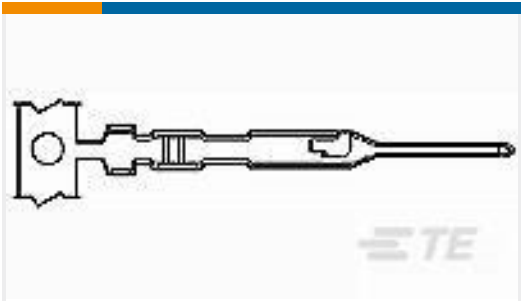
TE 产品编号1-104505-2 MTE PIN 22-26 AWG PLTD
