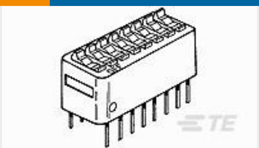
TE 产品编号3-435640-2 DIP SW 12 POSN AU
