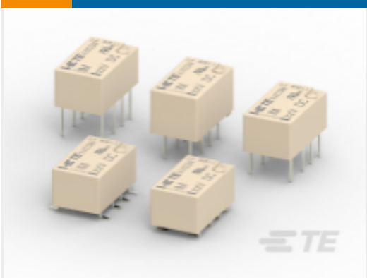
TE 产品编号1462039-2 标准信号继电器 2 Form C，2 CO 端子
