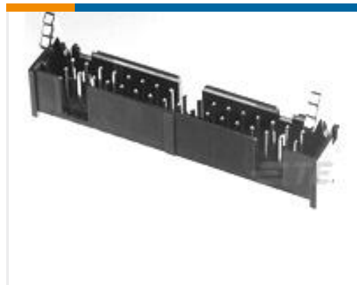
TE 产品编号1-1761606-0 IDC LOW PRO HDR 30P VERT LG LA
