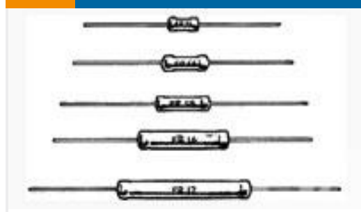
TE 产品编号1623746-9 ER74 180R 5% AMMO PK
