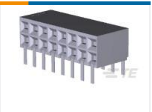
TE 产品编号1-5535512-8 16 MODII HORZ DR CE EESS .100
