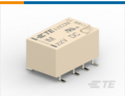
TE 产品编号1462041-7 信号继电器：1 Form A，1 NO 端子
