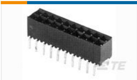
TE 产品编号1-829264-8 2X18P HV100 REC.CON.B/TE,6.2MM, NO KINK
