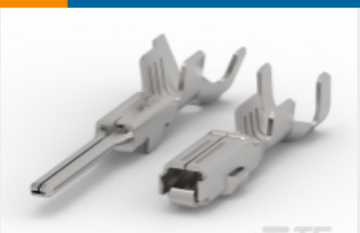
TE 产品编号1326031-9 1.5/2.8 连接器系统，母端和公端
