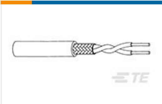
TE 产品编号287925-000 2530A0314-9
