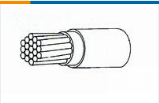
TE 产品编号712726-000 22759/43-12-4
