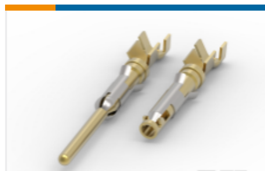
TE 产品编号163088-2 欧洲、中东和非洲类型 III 端子低型面
