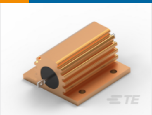
TE 产品编号1-1630012-9 功率电阻器：铝壳体，HSA
