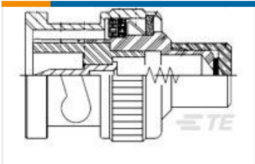
TE 产品编号1-1337463-0 BNC Plg Term 50Ohm Silver Pltd
