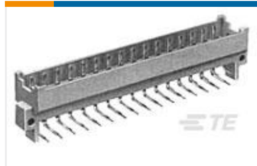
TE 产品编号2-164045-4 48P.IEC-F.MALE CONN
