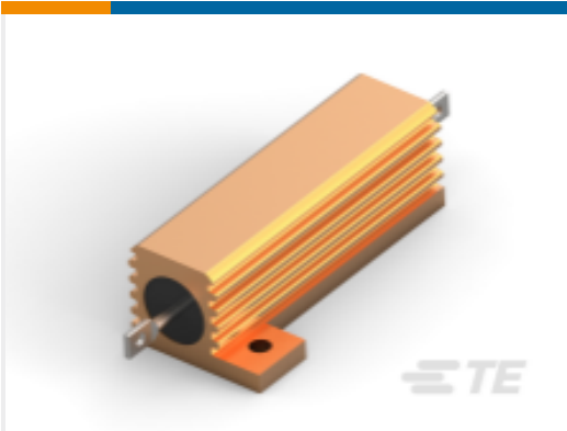
TE 产品编号1-1676814-4 功率电阻器：铝壳体，HSA
