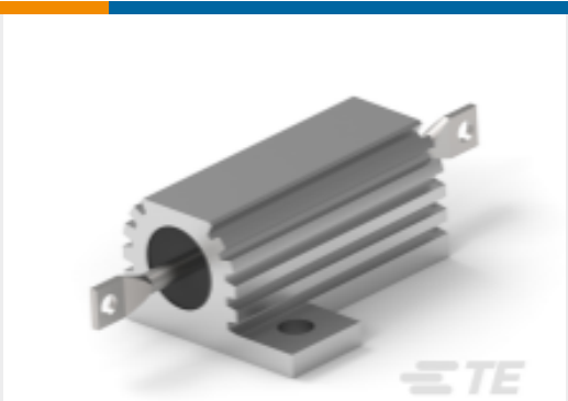
TE 产品编号1879075-1 功率电阻器：铝壳体，75 瓦特
