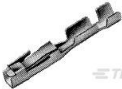
TE 产品编号126628-000 D-602-0173
