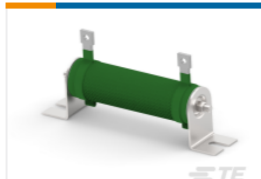
TE 产品编号 2-1879447-2 线绕电阻器：矿物，2.5 Kw
