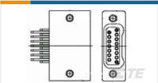
TE 产品编号5-1589483-5 STM037L2HN = SMT CONN
