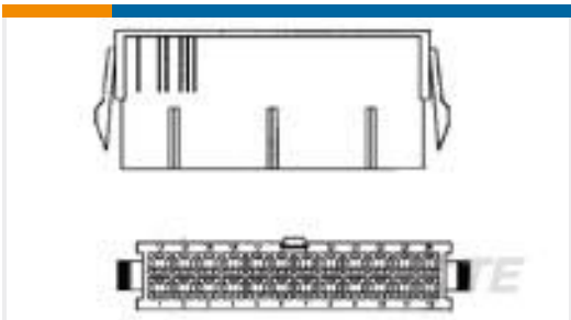
TE 产品编号2-1586018-4 24P PM PLUG VAL-U-LOK V0
