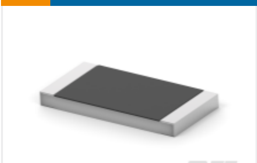
TE 产品编号1622820-4 SMD 功率电阻器：1 瓦特，3520 系列
